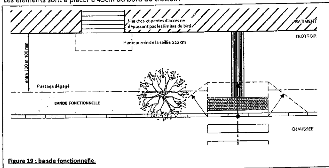
Figure 19 : bande fonctionnelle.
